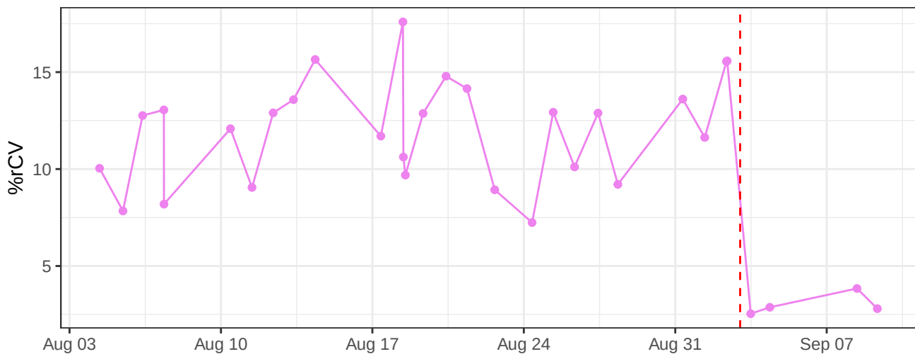
V540-A-% rCV
